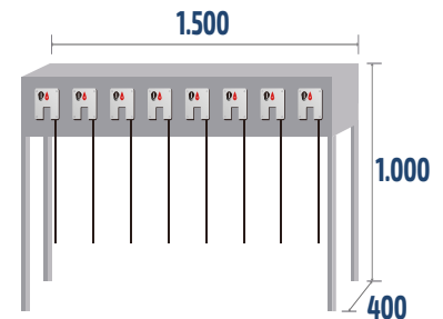
MA1500 COD: 90422 23,5kg · 0,10m 3 8 Gelddörse
